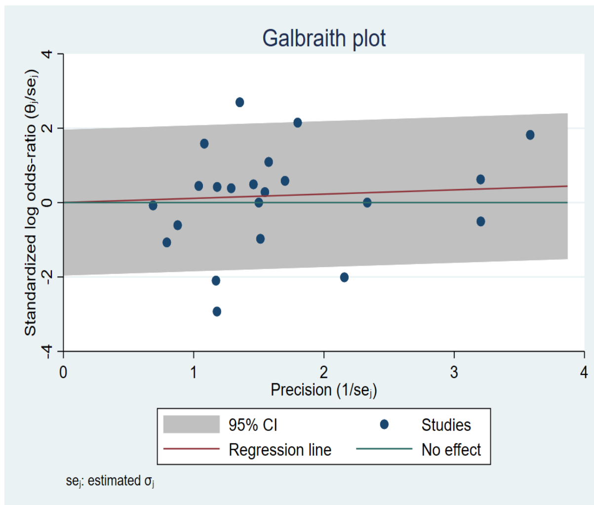
شکل ۴. نمودار Galbraith
