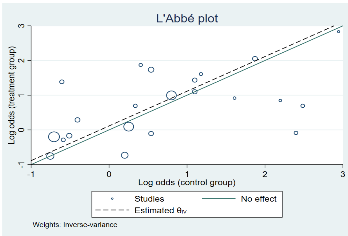
شکل ۵. نمودار L'Abbé
