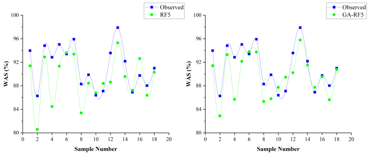
شکل ۸. مقایسه مقادیر WAS مشاهداتی و پیش‌بینی شده از مدل‌های RF5 و GA-RF5
