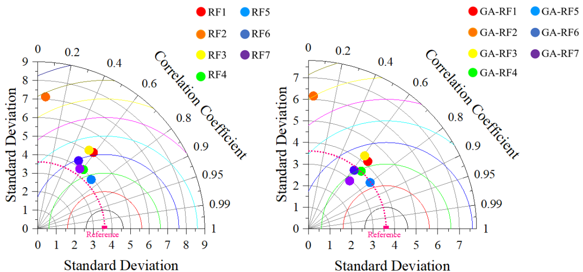
شکل ۵. دیاگرام‌های تیلور مدل‌ها
