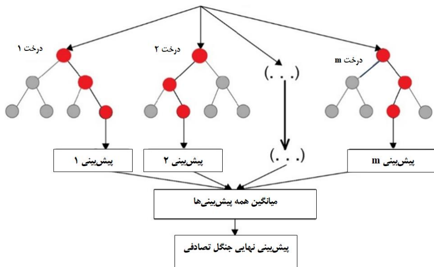
شکل ۲. روند کار RF (Zeini et al, 2023)
