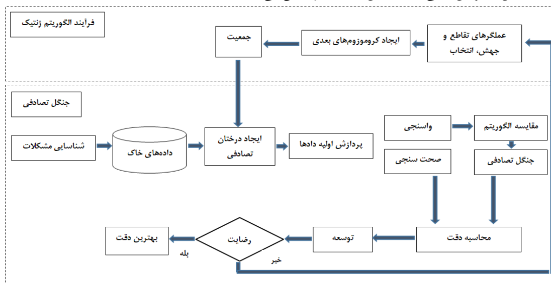
شکل ۳. نمودار مدل GA-RF (Ramdhani et al, 2023)
