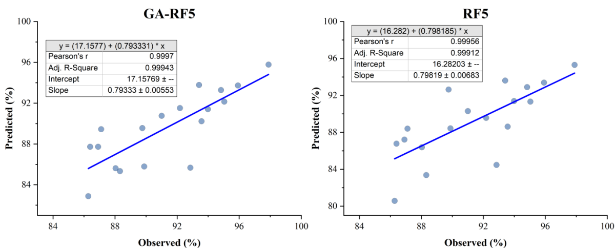
شکل ۷. پراکنش مقادیر WAS مشاهداتی و پیش بینی شده از مدل های RF5 و GA-RF5
