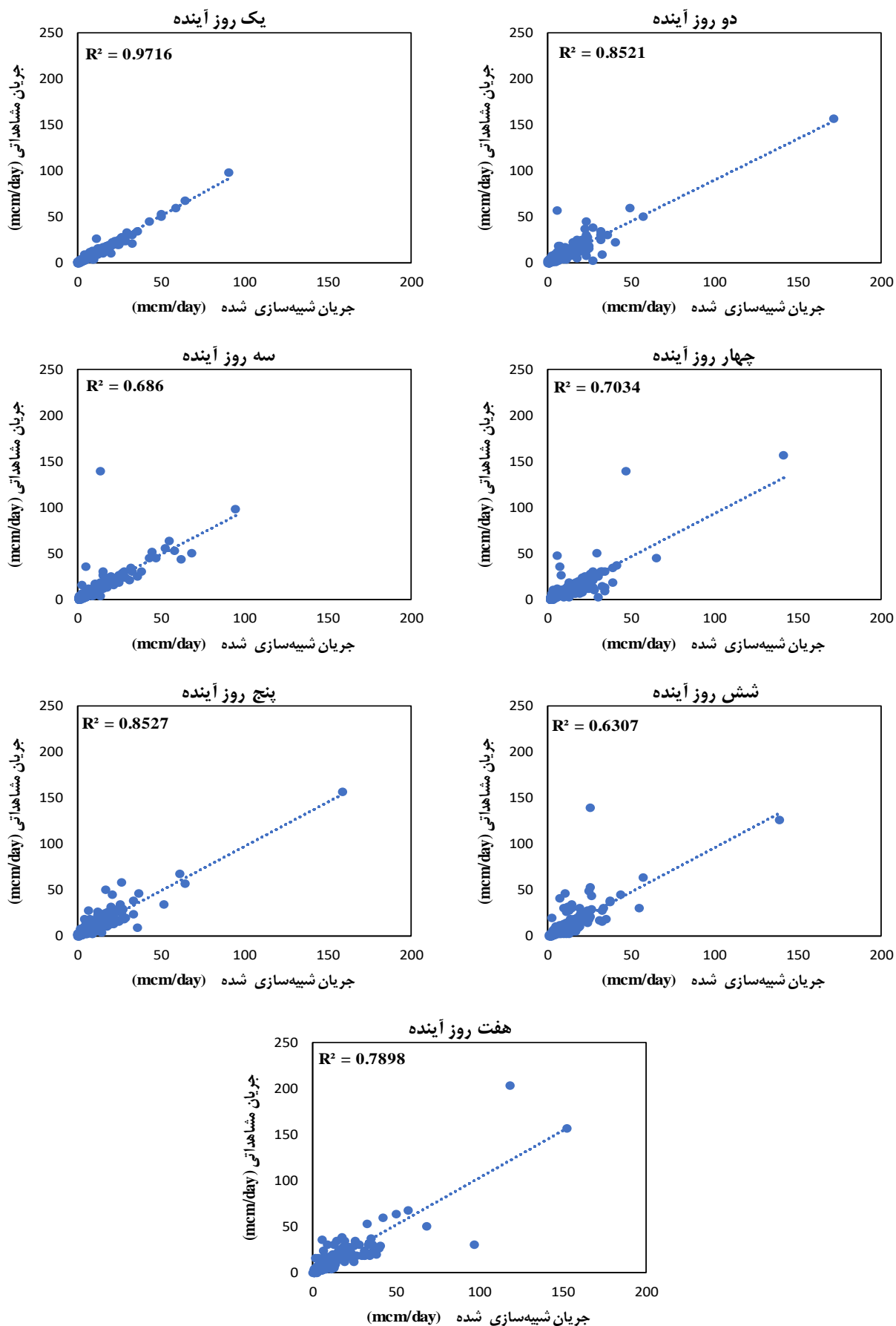
شکل ۶. مقایسه نتایج مدل LSTM با مقادیر مشاهداتی در مرحله آزمایش
