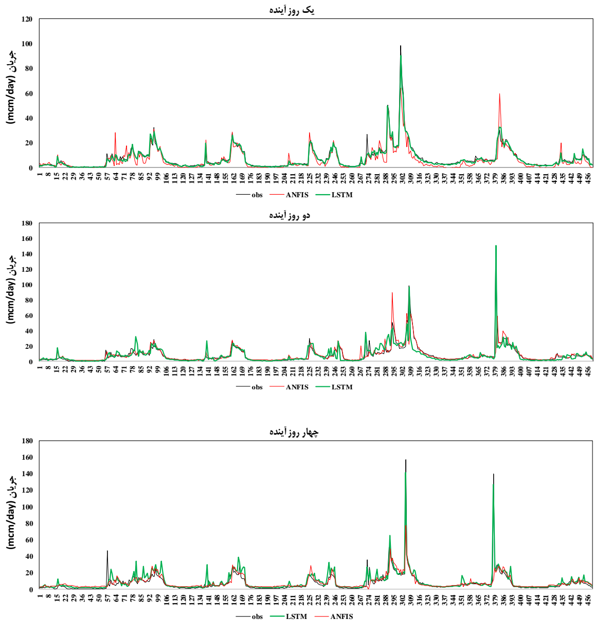
شکل ۷. جریان شبیه‌سازی شده توسط مدل‌های ANFIS و LSTM و جریان مشاهداتی در افق پیش‌بینی یک تا هفت روز آینده - مرحله آزمایش
