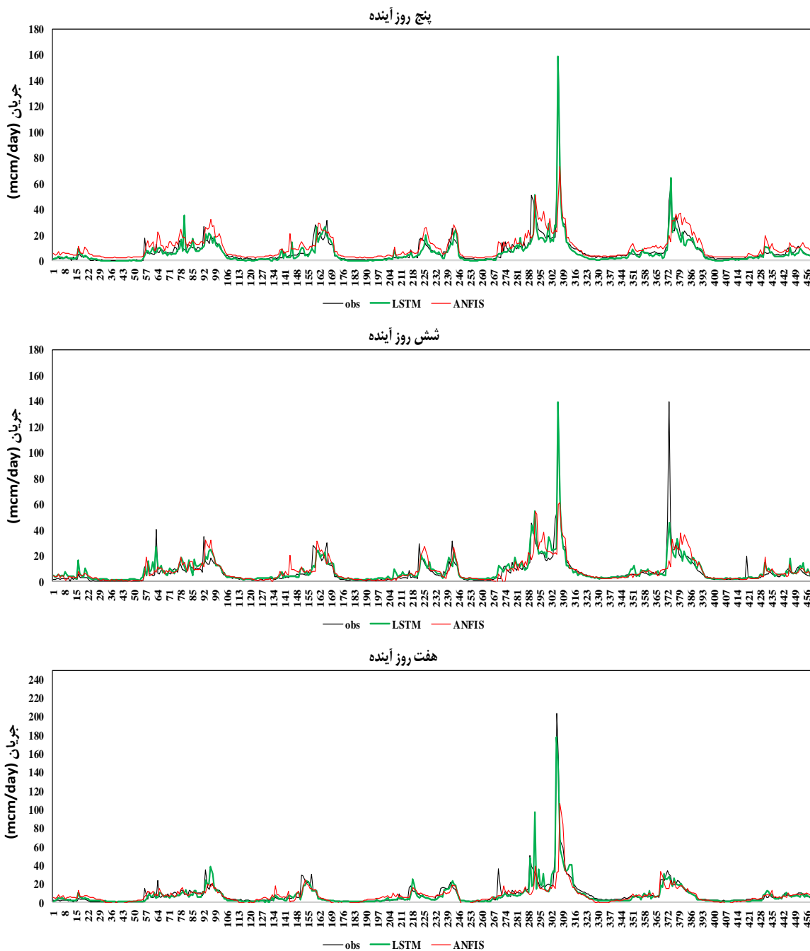
شکل ۷. جریان شبیه‌سازی شده توسط مدل‌های ANFIS و LSTM و جریان مشاهداتی در افق پیش‌بینی یک تا هفت روز آینده - مرحله آزمایش
