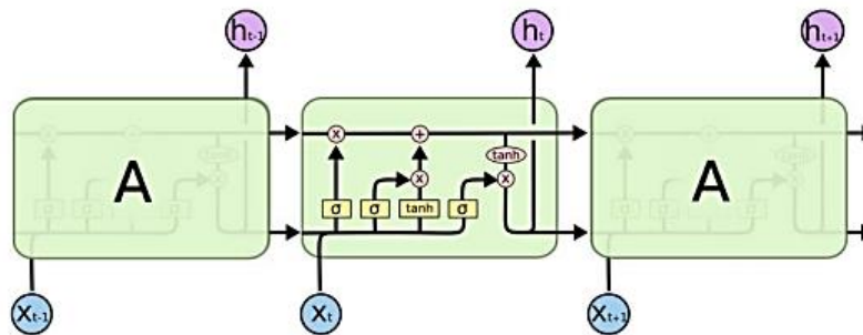
شکل ۳. ساختار شبکه‌های بازگشتی LSTM (ساختار تکرارشونده و چهار لایه‌ای) (Olah 2015)
