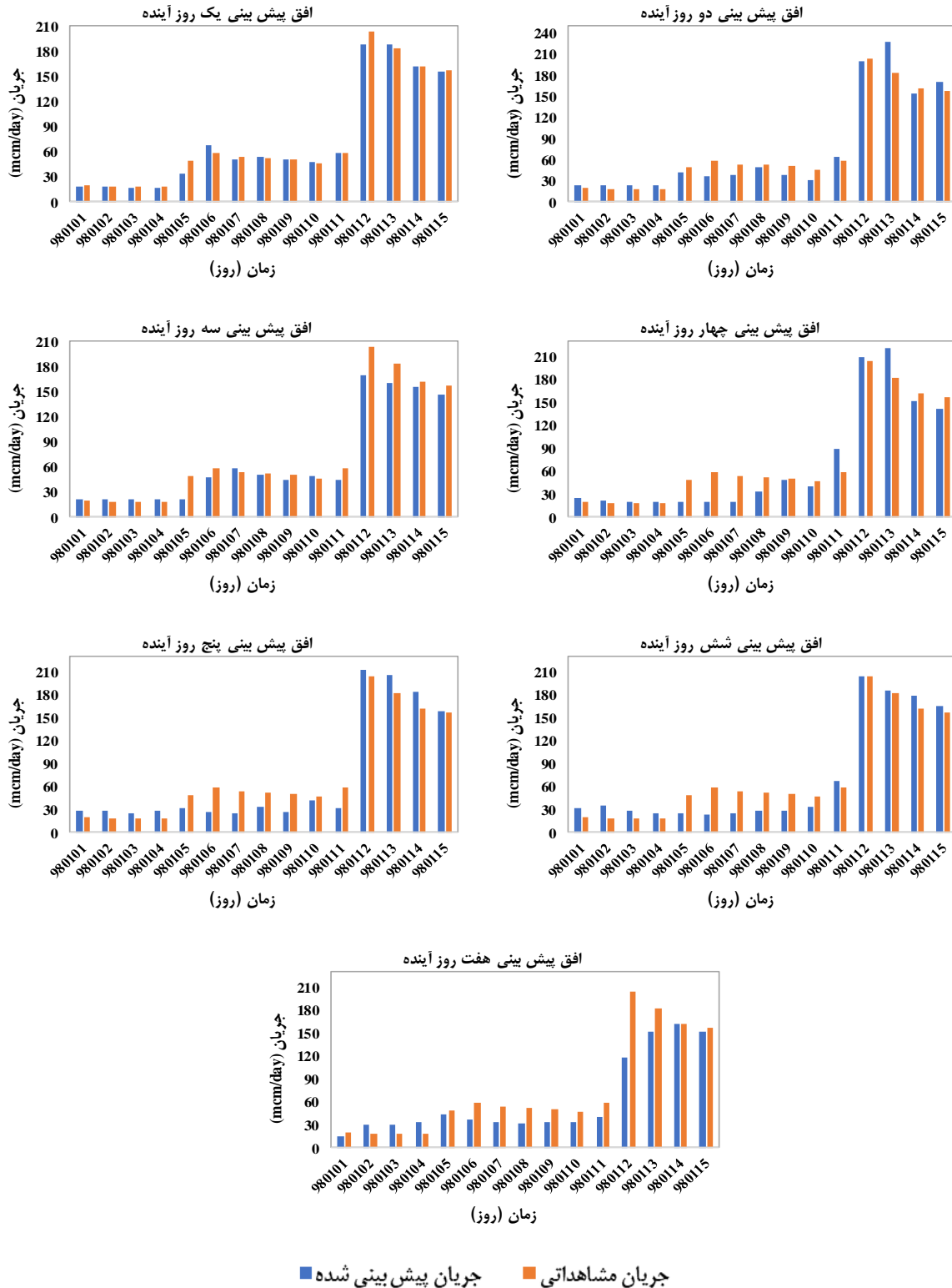
شکل ۸. مقایسه مقادیر پیش‌بینی‌شده مدل LSTM با مقادیر ثبت‌شده جریان ورودی به سیمره در سیلاب ۹۸
