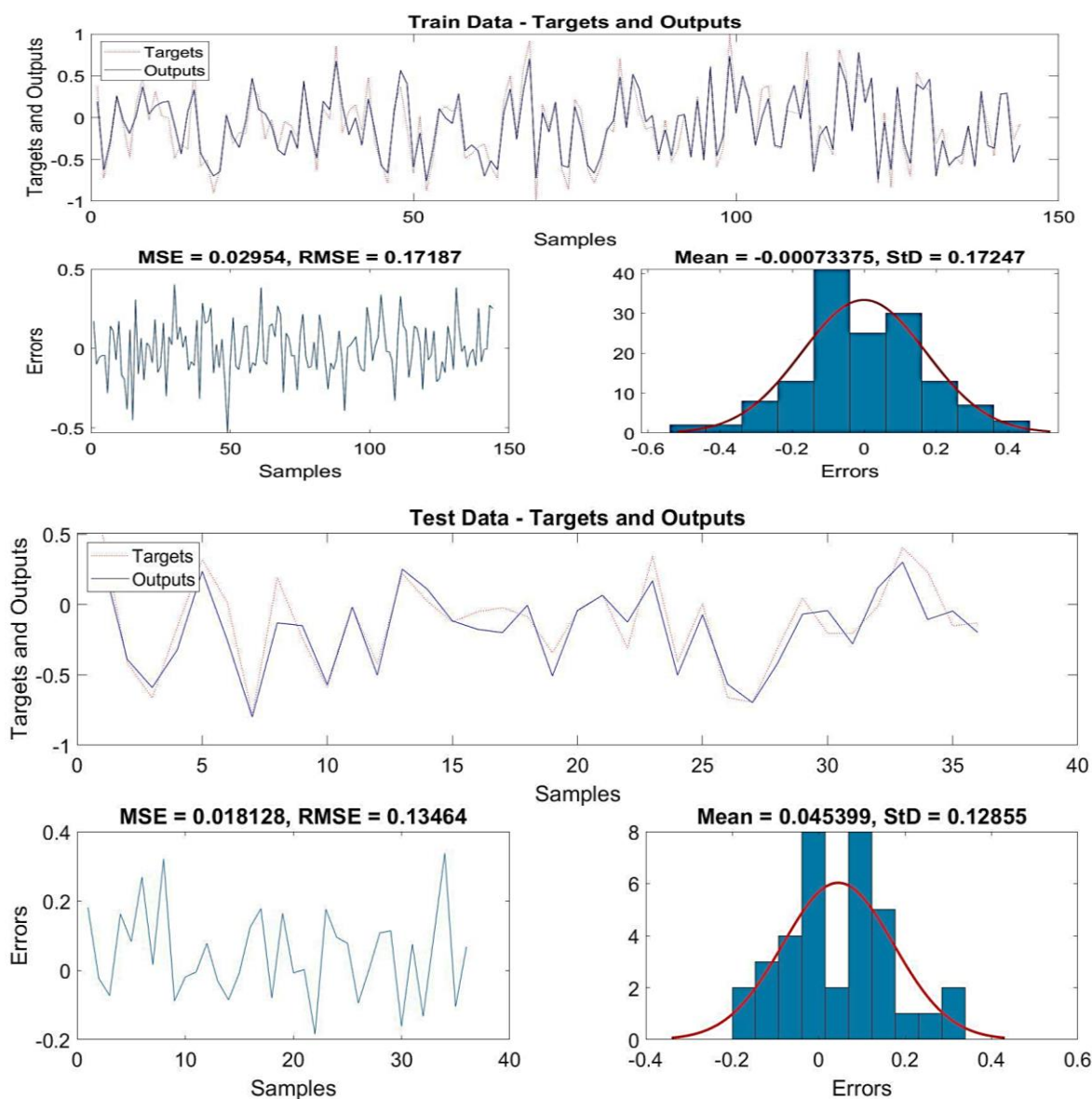
شکل ۵. سری زمانی مقادیر پیش‌بینی شده تراز آب زیرزمینی بر اساس مدل برتر (ICA-ANN) در مقایسه با داده‌های مشاهده‌ای در مراحل آموزش و تست در نقطه مطالعاتی ۲
