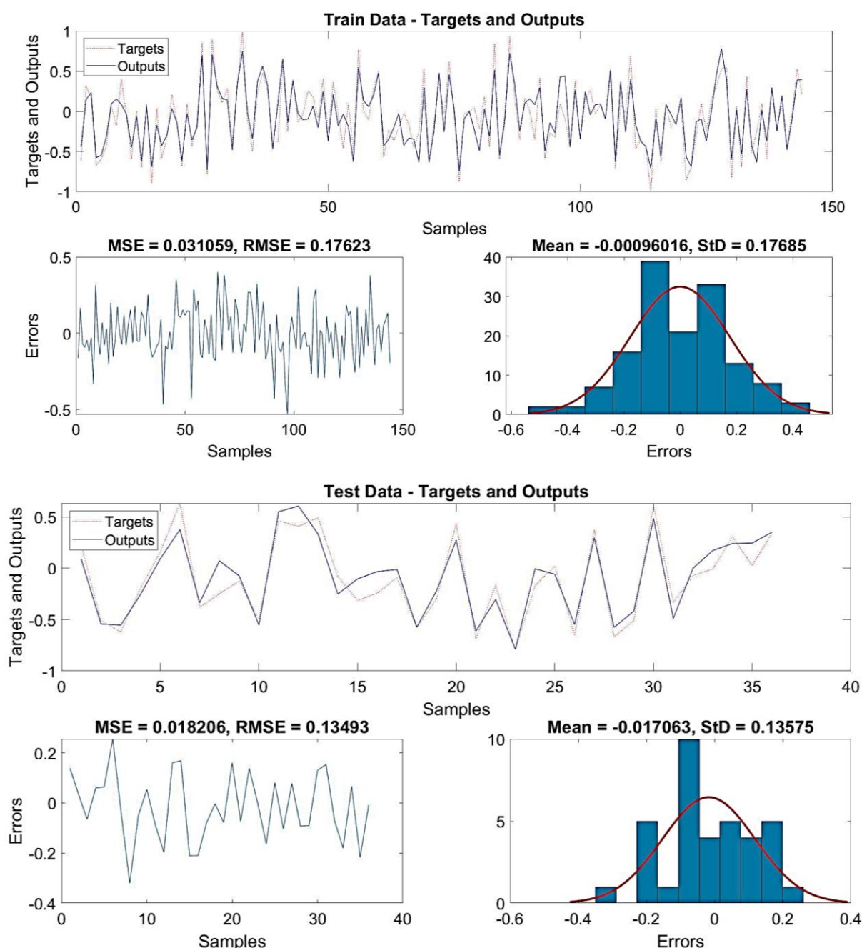
شکل ۶. سری زمانی مقادیر پیش‌بینی شده تراز آب زیرزمینی بر اساس مدل برتر (ICA-ANN) در مقایسه با داده‌های مشاهده‌ای در مراحل آموزش و تست در نقطه مطالعاتی ۵
