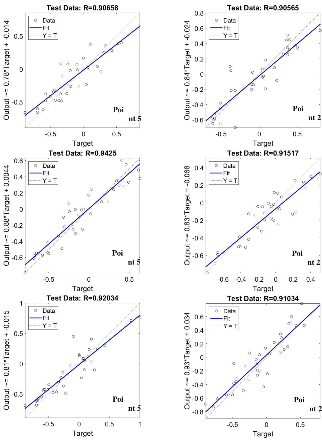
شکل ۴. نمایش گرافیکی پراکنده‌گی نقاط در اطراف خط Y=X و مقدار مجذور ضریب همبستگی برای انتخاب بهترین مدل هوش مصنوعی در مرحله تست مدل‌سازی در نقاط مطالعاتی ۲ و ۵
