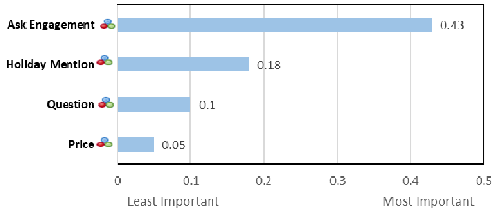
شکل ۵. نمودار تأثیر فیلدها بر خروجی گفت‌وگوهای سایر
