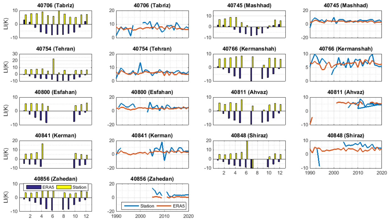
شکل ۴: نمودار میله‌ای ماهانه و سری زمانی شاخص LI برای نه ایستگاه جو بالا. نمودار میله‌ای در بازه زمانی که هر دو نوع داده مشاهداتی و ERA5 در دسترس بوده‌اند ترسیم شده است، در حالی که برای ترسیم سری زمانی، کل داده‌های در دسترس ERA5 و مشاهداتی به‌طور مستقل استفاده شده است.
