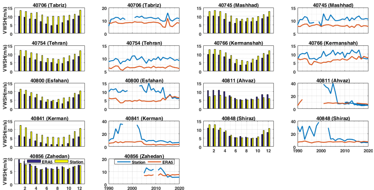
شکل ۲. نمودار میله‌ای ماهانه و سری زمانی پارامتر VWSH-3000 برای نه ایستگاه جو بالا. نمودار میله‌ای در بازه زمانی که هر دو نوع داده مشاهداتی و بازتحلیل ERA5 در دسترس بوده‌اند، ترسیم شده است؛ در حالی که برای ترسیم سری زمانی کل داده‌های در دسترس ERA5 و مشاهداتی به‌طور مستقل استفاده شده است.
