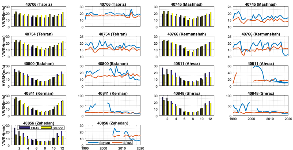
شکل ۳. نمودار میله‌ای ماهانه و سری زمانی پارامتر VWSH-6000 برای نه ایستگاه جو بالا. نمودار میله‌ای در بازه زمانی که هر دو نوع داده مشاهداتی و بازتحلیل ERA5 در دسترس بوده‌اند ترسیم شده است، در حالی که برای ترسیم سری زمانی، کل داده‌های در دسترس ERA5 و مشاهداتی هر یک به‌طور جداگانه استفاده شده است.
