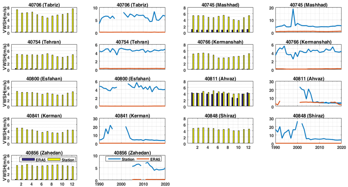
شکل ۱. نمودار میله‌ای ماهانه و سری زمانی پارامتر WWSH-1000 برای نه ایستگاه جو بالا. نمودار میله‌ای در بازه زمانی که هر دو نوع داده مشاهداتی و بازتحلیل ERA5 در دسترس بوده‌اند ترسیم شده است، در حالی که برای ترسیم سری زمانی کل داده‌های در دسترس ERA5 و مشاهداتی به‌طور مستقل استفاده شده است.
