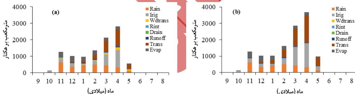
شکل ۵. شبیه‌سازی متغیرهای بیلان آب (شامل بارندگی، آبیاری، تبخیر، تعرق، زهکشی عمقی، رواناب، تعرق علف‌های هرز و برگاب) برای یک هکتار گندم آبی در شرایط «مزارع کشاورزان» (a) و «پتانسیل» (b) در پهنه آگروکولوژیک 6002Shrz (ایستگاه هواشناسی شیراز) در ماه‌های مختلف سال میلادی (بر حسب مترمکعب در هکتار). شبیه‌سازی‌ها بر اساس اطلاعات هواشناسی سال‌های ۲۰۱۱ تا ۲۰۲۱ میلادی انجام شده است. چنین برآوردهایی برای ۳۵ گیاه مهم برای سایر پهنه‌ها و نیز کل استان قابل تهیه است.
