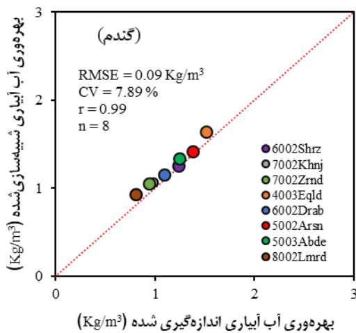
شکل ۶ مقایسه برآوردهای سامانه از حجم آب آبیاری ( m^3/Ha )، عملکرد ( Kg/Ha ) و بهره‌وری آب آبیاری ( Kg/m^3 ) برای گیاه گندم و جو در پهنه‌های همگن تعریف شده در این مطالعه در شرایط واقعی کشاورزان در برابر مقادیر اندازه‌گیری شده توسط عباسی و همکاران (۱۴۰۱). اندازه‌گیری‌ها از تعدادی از مزارع کشاورزان برای گیاه گندم در سال زراعی ۱۳۹۹-۱۴۰۰ و برای گیاه جو در سال زراعی ۱۳۹۵-۱۳۹۶ انجام گرفته است که در اینجا از معدل آن‌ها استفاده شده است. بنابراین، هر نقطه معادل پارامتر شبیه‌سازی شده توسط مدل در شرایط کشاورزان در برابر معدل پارامتر واقعی اندازه‌گیری شده توسط عباسی و همکاران (۱۴۰۱) در مزارع کشاورزان در سال مورد نظر است.
