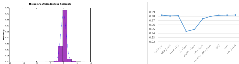
نمودار ۲. حساسیت‌سنجی مدل رگرسیون لجستیک به حذف متغیرهای مستقل شکل ۱۲. بافت‌نگار مقادیر استاندارد شده باقی‌مانده‌های مدل رگرسیون حداقل مربعات (OLS)
