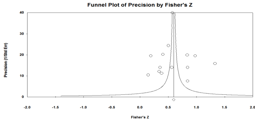
نمودار ۱. بررسی میزان همگنی و ناهمگنی پژوهش
