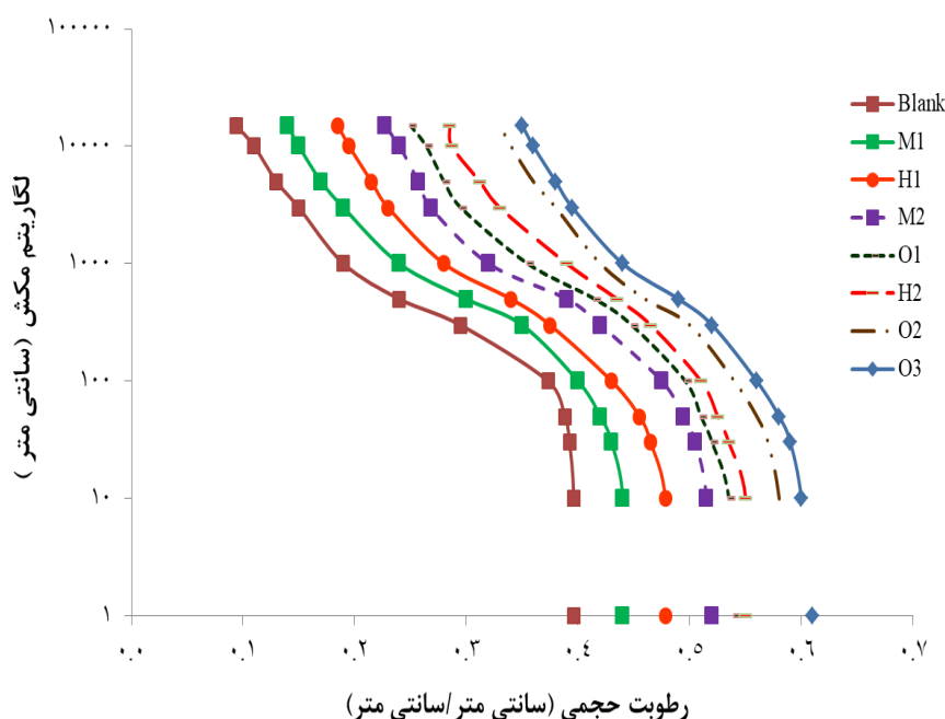
شکل ۴. منحنی‌های نگهداری آب خاک برای تیمارهای مختلف پس از چهار ماه در کرت‌های فرسایشی
