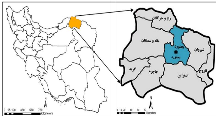
شکل ۲. موقعیت شهر بجنورد در کشور و استان خراسان شمالی، مأخذ: موسسه آموزش عالی اشراق، ۱۳۹۸: ۱۸۰ و ۱۸۱
