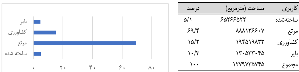
جدول ۵. مساحت و درصد هر کاربری در سال ۲۰۲۱؛ شکل ۷. درصد سهم هر یک از کاربری‌ها در سال ۲۰۲۱
