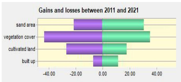
شکل ۹. آنالیز تغییرات بین سال‌های ۲۰۱۱ تا ۲۰۲۱ (برحسب کیلومتر مربع)
