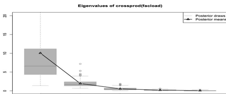
نمودار ۱. مقادیر مشخصه و شناسایی تعداد عوامل نهفته
