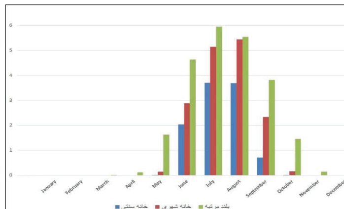
شکل ۸. نمودار مقایسه‌ای پایه‌ای میزان مصرف سالانه انرژی سرمایه‌شناسی و تحلیل بار سرمایه‌شناسی مربوط به سه بنای ب.م.۱، ب.م.۲، ب.م.۳ بر اساس تحلیل نرم‌افزاری انرژی پلاس
