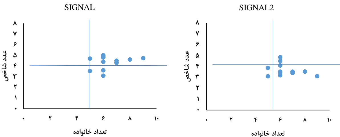
شکل ۴. نتایج شاخص سیگنال از ۴ ایستگاه در فصول نمونه‌برداری از رودخانه مادرسو
