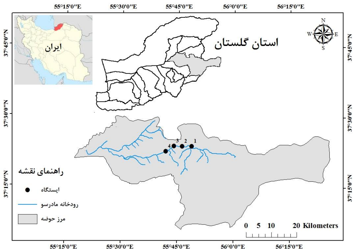
شکل ۱. ایستگاه‌های نمونه‌برداری از رودخانه مادرسو، استان گلستان
