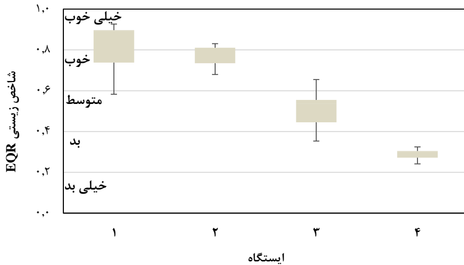
شکل ۵. نمودار باکس ویسکر برای طبقه‌بندی ایستگاه‌ها در طی فصول نمونه‌برداری بر اساس شاخص زیستی EQR
