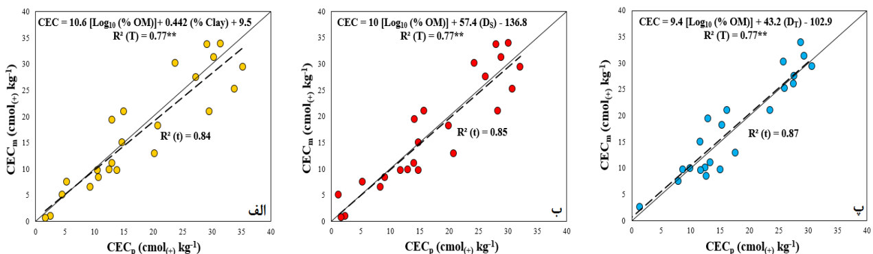
شکل ۷- پراکنش مقادیر ظرفیت تبادل کاتیونی اندازه گیری و برآورد شده حول خط ۱:۱ برای ارتباط رگرسیونی مقادیر ظرفیت تبادل کاتیونی (CEC) با الف) لگاریتم (در پایه ۱۰) درصد ماده آلی ( Log_{10} [OM (\%)] ) و رس (Clay)، ب) لگاریتم (در پایه ۱۰) درصد ماده آلی و بعد فرکتالی سپاسخواه و تافته ( D_s ) و پ) لگاریتم (در پایه ۱۰) درصد ماده آلی و بعد فرکتالی تایلر و ویت کرفت ( D_T ). CEC_p و CEC_m به ترتیب نشان دهنده مقادیر ظرفیت تبادل کاتیونی اندازه گیری شده و برآورد شده هستند.
