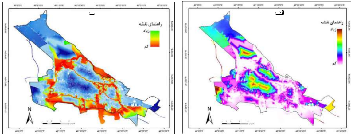
شکل ۷. (الف) نقشه فواصل وزن دار هزینه (ب) موزاییک مناطق اصلی و کریدورهای حداقل هزینه
