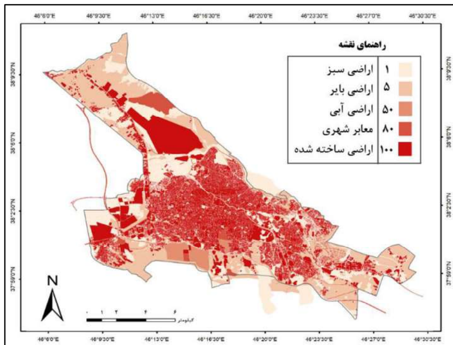
شکل ۶. نقشه لایه مقاومت / هزینه برای هر کدام از کاربری اراضی شهر تبریز، اعداد درج شده در نقشه در واقع میزان مقاومت هر کدام از کاربری اراضی را نشان می‌دهند که بر اساس تحلیل‌های نویسنده‌گان به دست آمده‌اند (مأخذ: نگارندگان)
