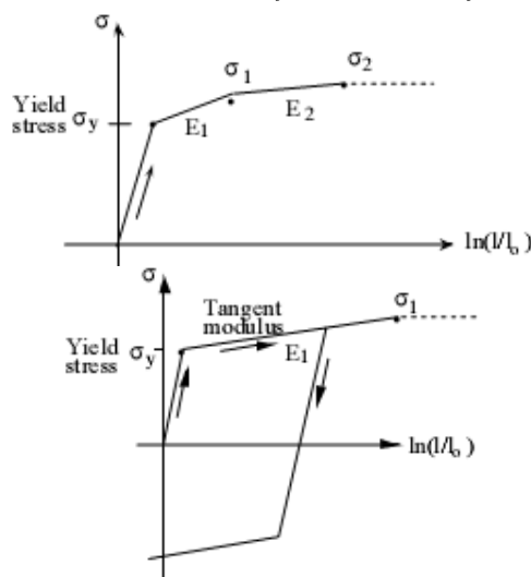
شکل ۲: مدل‌سازی رفتار الاستوپلاستیک مواد.
