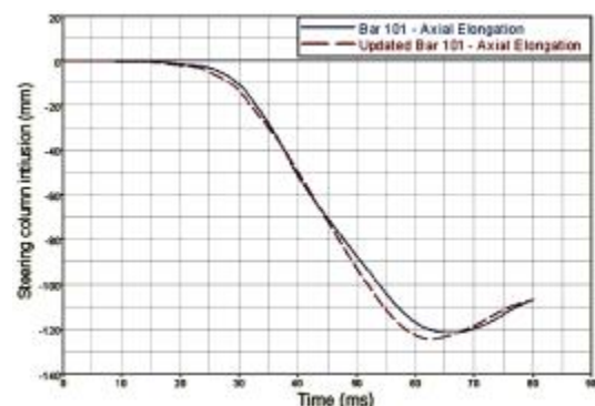
شکل ۱۸: مقایسه میزان نفوذ ستون فرمان به اتاقک سرنشین در راستای افقی.
