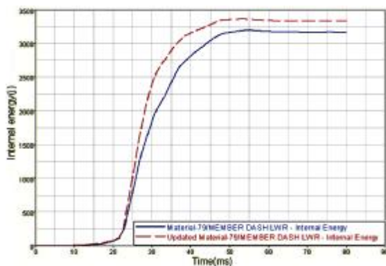
شکل ۱۱: مقایسه میزان جذب انرژی ورق داشبورد قبل و پس از تغییر ضخامت.
