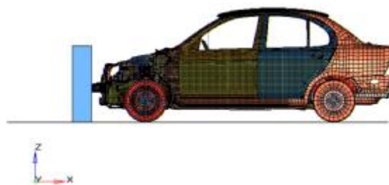
شکل ۱. مدل ساخته شده جهت تحلیل برخورد طولی.
