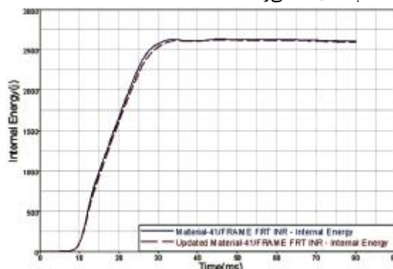
شکل ۱۷: مقایسه میزان انرژی جذب شده تیر طولی (قاب) جلو قبل و بعد از تغییر ضخامت.
