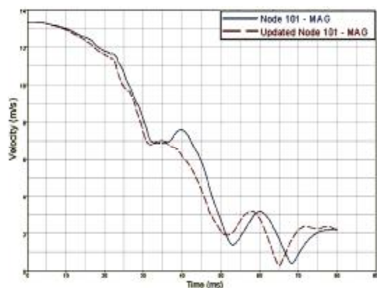
شکل ۱۶: مقایسه سرعت محل نصب صندلی راننده برای دو خودروی دارای سپر فلزی و سپر کامپوزیتی.
