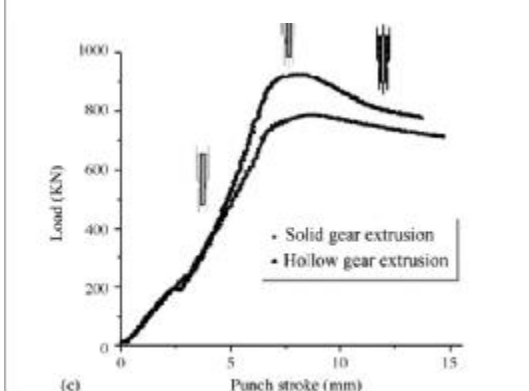
شکل ۹: نتایج آزمایش انجام شده برای الف: چرخ دنده ساده توخالی و ب: توپر با مشخصات شکل (۵) [۲].
