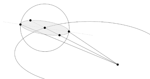
شکل ۱۰. ساختار کمابیش مجسم فلک تدویر در مدل عرض در مجسطی
