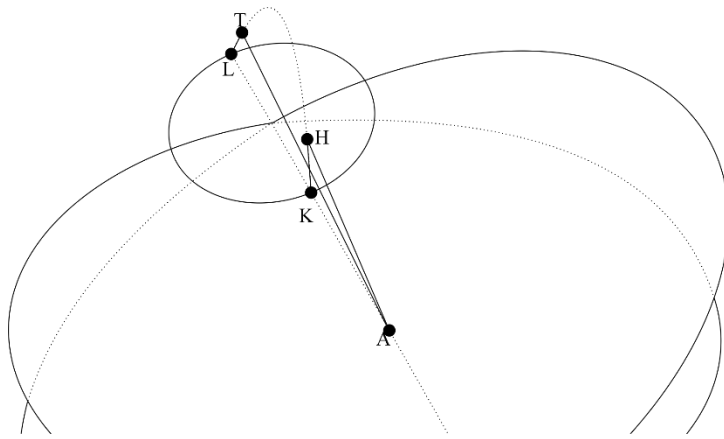
شکل ۷. تشکیل کمان زاویه میل تدویر سیارات داخلی در چشم رصدگر (برگرفته از یاوری، ص ۱۹)
