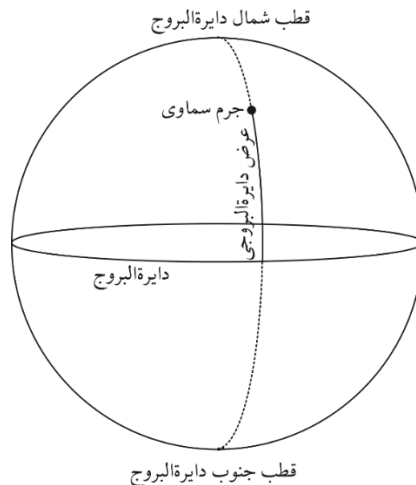
شکل ۳. عرض دایرة البروجی
