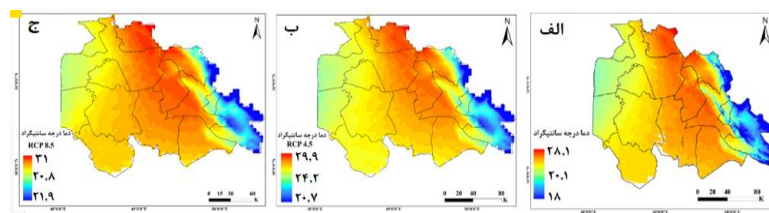
شکل ۲. الف) توزیع فضایی میانگین دمای منطقه تحقیق در دوره کنونی؛ ب) توزیع فضایی میانگین دمای سال ۲۰۷۰ تحت سناریوی RCP4.5؛ ج) توزیع فضایی میانگین دمای سال ۲۰۷۰ تحت سناریوی RCP8.5.
