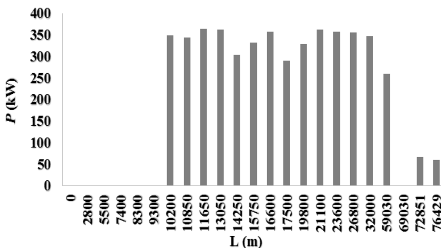
شکل ۹. تغییرات پتانسیل توان (P) طی خط انتقال گاوشان به تصفیه‌خانه شهید نظری
