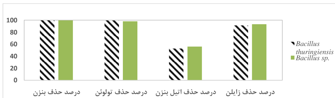
شکل ۱- درصد حذف BTEX توسط باکتری‌های Bacillus sp. و Bacillus thuringiensis
