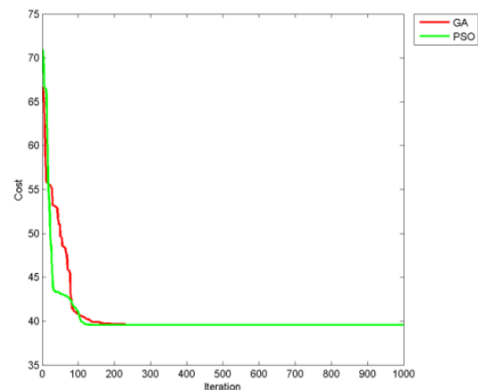
شکل ۴. مقایسه نمودار برازندگی الگوریتم ازدحام ذرات و ژنتیک
