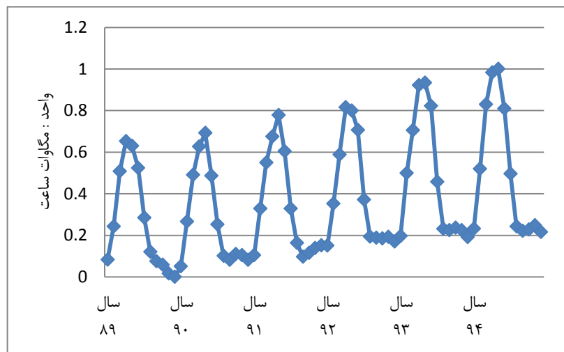
شکل ۲. کل نیاز مصرف ماهانه نرمال شده شبکه برق ایران در طول فروردین‌ماه سال ۱۳۸۹ تا اسفندماه سال ۱۳۹۴
