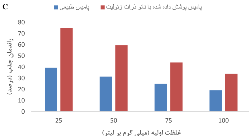
شکل ۶. نمودار اثر زمان تماس بر روی راندمان حذف نیترات توسط سنگدانه های پامیس طبیعی و اصلاح شده در شرایط بهینه (A)، تاثیر مقدار غلظت‌های اولیه متفاوت بر ظرفیت جذب نیترات در شرایط بهینه (B) و تاثیر مقدار غلظت‌های اولیه متفاوت بر راندمان حذف نیترات در شرایط بهینه (C)
