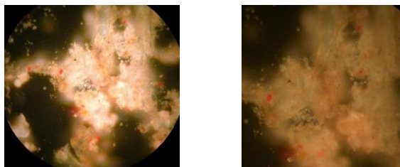
تصویر ۲۰: تصاویر میکروسکوپی رنگ صورتی که در آن استفاده از دو رنگ قرمز شنگرف و سفید هانتیت به خوبی مشهود است، بزرگنمایی X400
