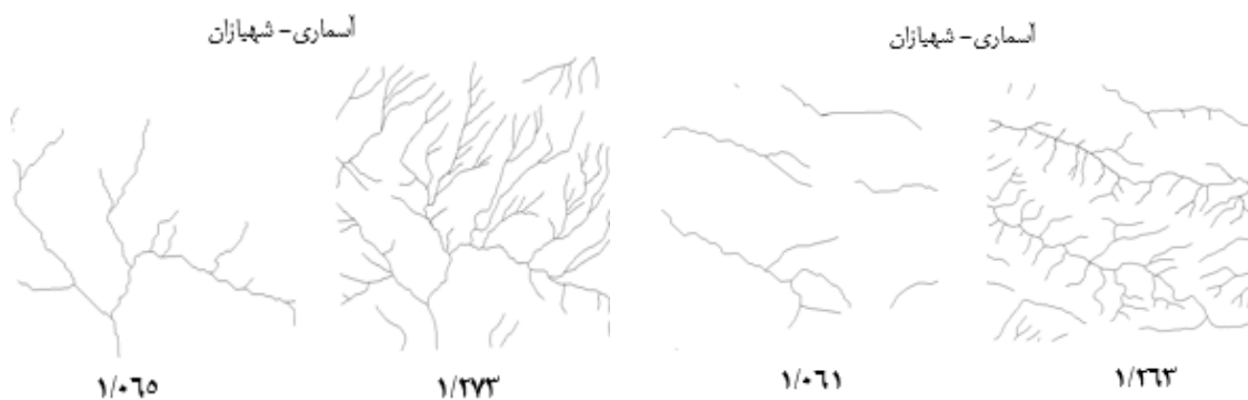
شکل ۴. بُعد فراکتال نمونه‌ای از شبکه هیدروگرافی سازند آسماری - شهپازان قبل و پس از اصلاح شبکه هیدروگرافی
