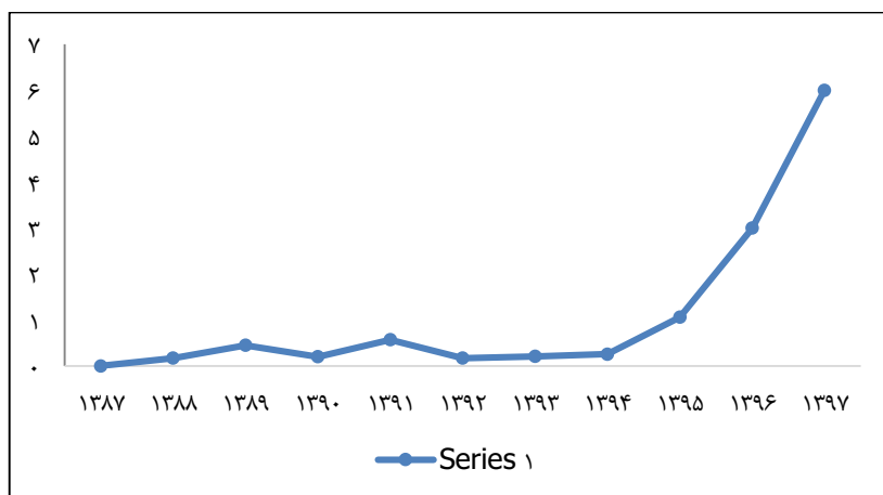
شکل ۲. نمودار نسبت پژوهش‌های کیفی و آمیخته به پژوهش‌های کمی
