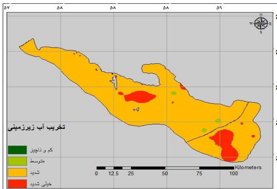
شکل ۶. نقشه تخریب بیابان‌زایی آبخوان مطالعه‌شده
