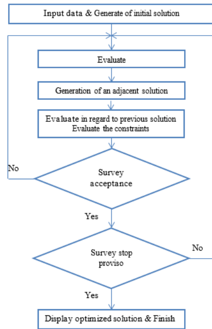
Fig. 1 SA flowchart
