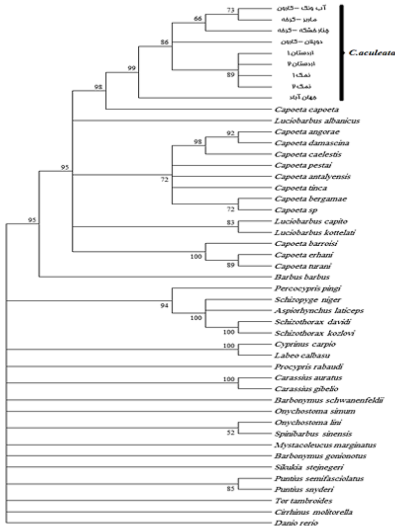
شکل ۳ - درخت شجره شناسی ترسیم شده بر اساس روش الحاق همسایگی (NJ) برای توالی‌های به دست آمده در این بررسی و توالی‌های گرفته شده از بانک ژن اعدادی که کنار گره‌ها مشاهده می‌شوند، ضریب صحت آزمون بوسترپ با ۱۰۰۰ تکرار هستند.
