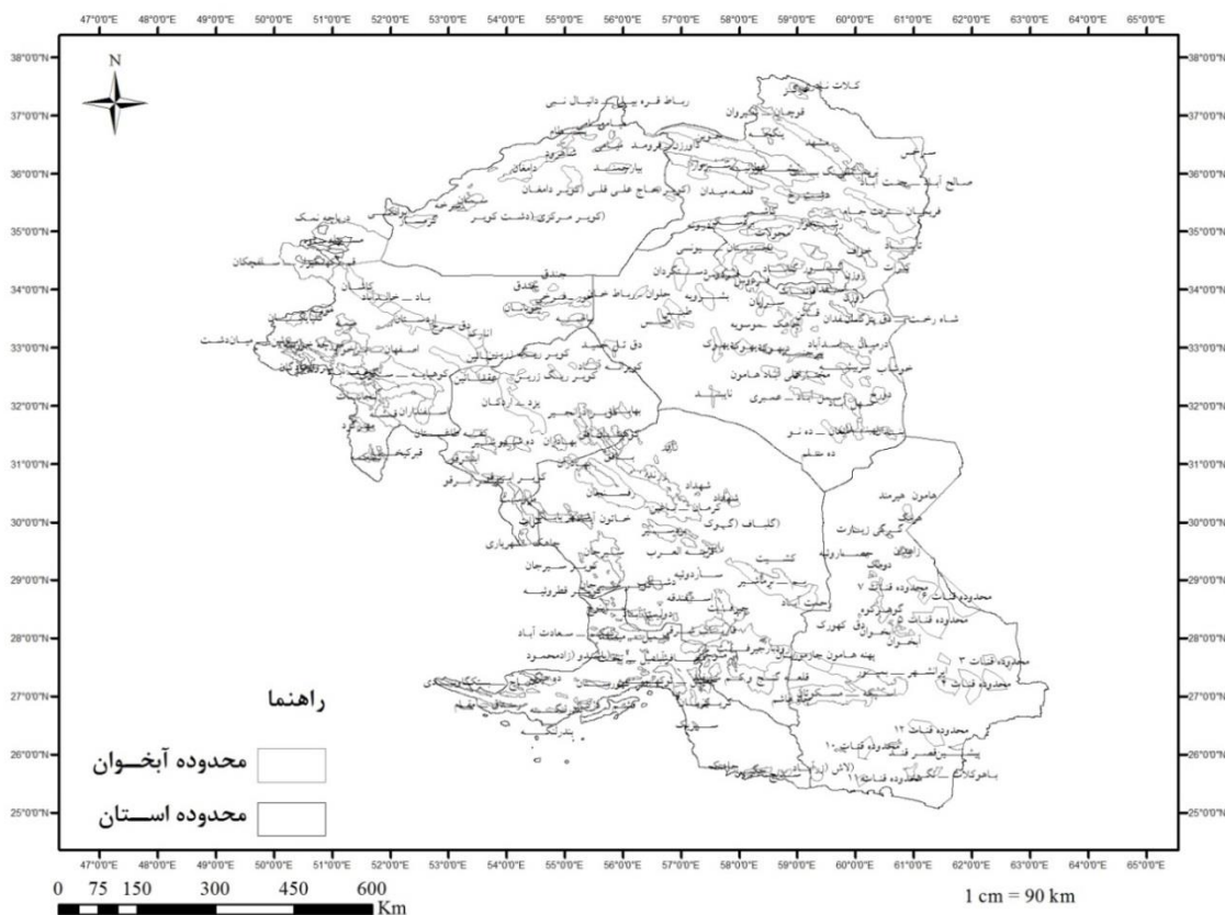
شکل ۱۰. محدوده مطالعاتی تحقیق
