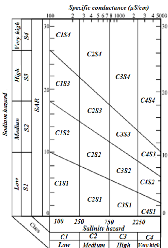
شکل ۲۰. دیاگرام ویلکوکس جهت تعیین کیفیت آب کشاورزی
