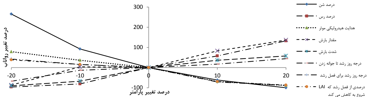
شکل ۸. آنالیز حساسیت مدل WEPP (رگبار بهار - رواناب - پلات ۱۶)
