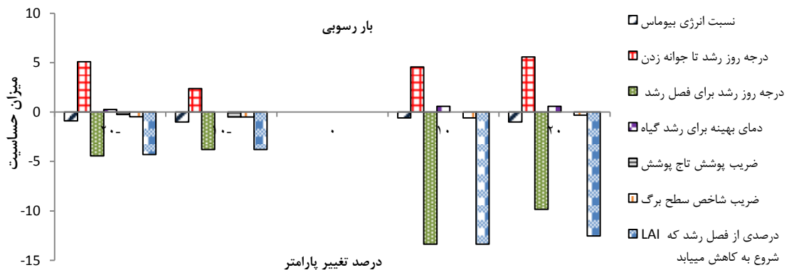
شکل ۶. آنالیز حساسیت فایل گیاه مدل WEPP (رگبار بهاره- پلات ۱۶)
