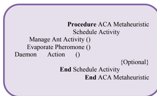
شکل ۱. ساختار کلی الگوریتم کلونی مورچگان منبع: سپهری و رحیمی مقدم (۱۳۸۶)
