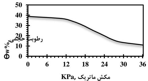
شکل ۴. منحنی مشخصه خاک جهت مقایسه مقادیر ضریب نسبی نفوذپذیری خاک در شکل ۳
