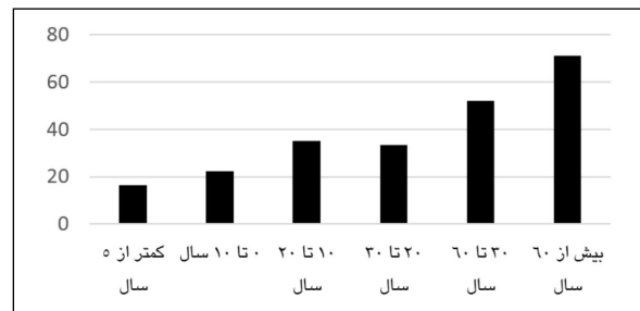
نمودار ۴- سرانه مصرف انرژی عملکردی (MJ) بر اساس عمر بنا.
