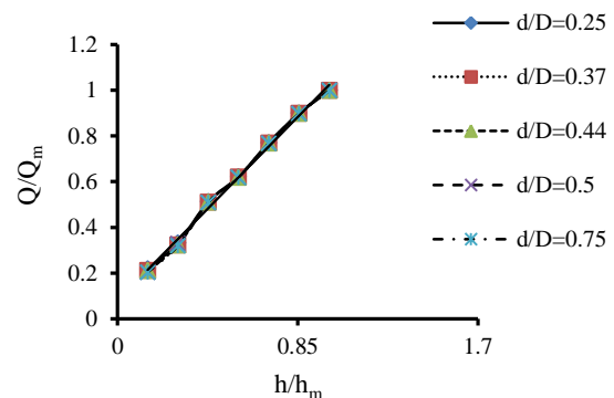
شکل ۵. اثر تراز آب بالادست بر میزان نشت
