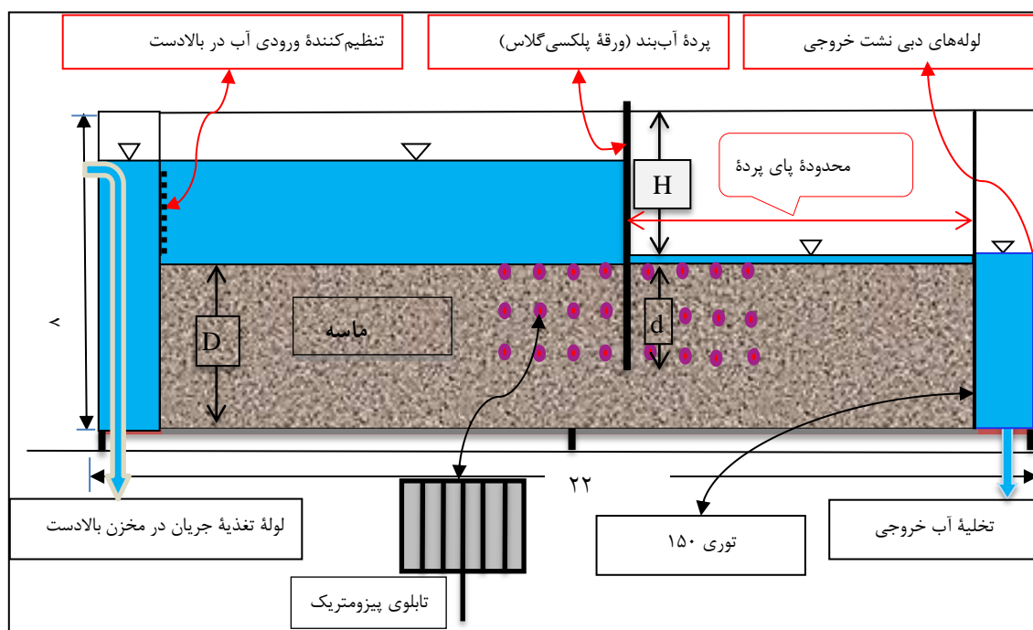
شکل ۲. طرح شماتیک مدل آزمایشگاهی
