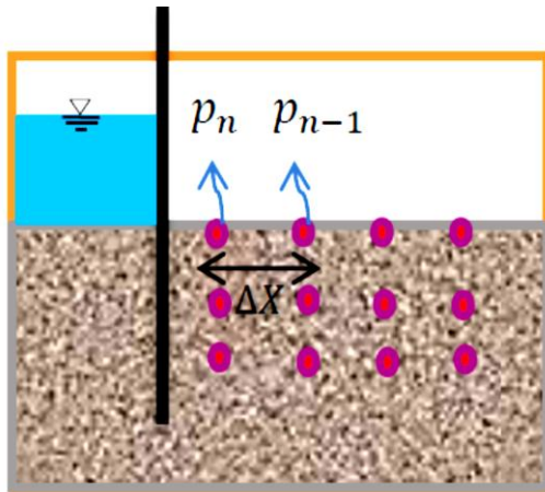
شکل ۷. مقطعی از پیزومترهای پایین دست
