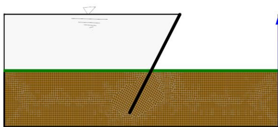
شکل ۲۰. شبکه‌بندی مدل عددی برای پرده آب‌بند مایل
