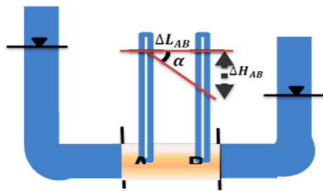
شکل ۶. شیب هیدرولیکی
