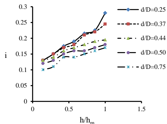
شکل ۹. تغییرات گرادیان هیدرولیکی نسبت به تراز آب بالادست
