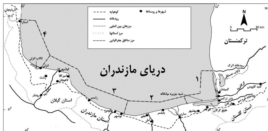
شکل ۶. محدوده جنوبی دریای مازندران و چهار بخش در نظر گرفته شده برای ژئومورفولوژی ساحل و محدوده آبی نزدیک به ساحل (برگرفته از: نادری بنی و همکاران، ۲۰۱۳: ب: شکل ۳)
