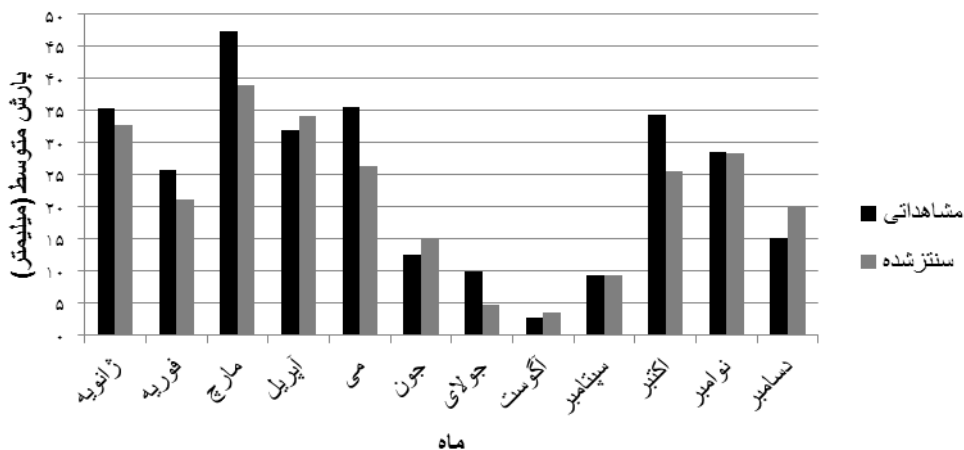
شکل ۴. مقایسه مقادیر متوسط ماهانه بارش مشاهداتی و سنتر شده از HadCM3-A2 (ایستگاه اردبیل - دوره ۱۳۵۵ - ۱۳۸۰)
