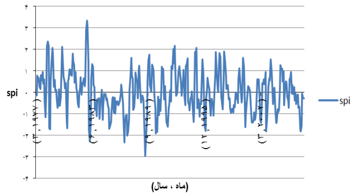
شکل ۵. نمودار نمایه استاندارد شده بارش ۳ ماهه در دوره مشاهداتی
