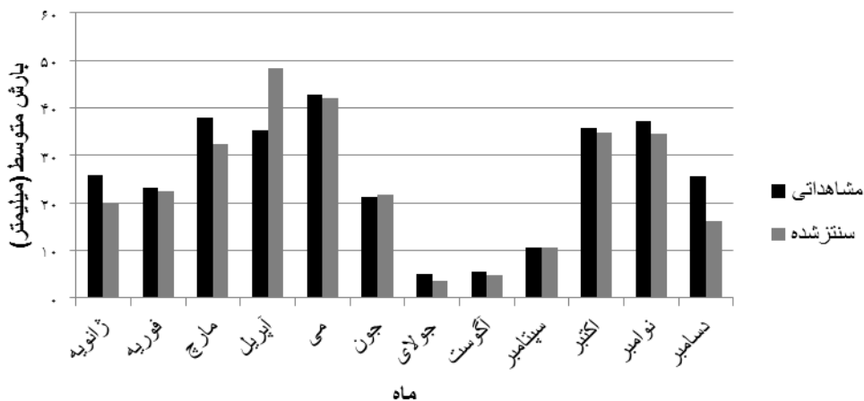
شکل ۳. مقایسه مقادیر متوسط ماهانه بارش مشاهداتی و سنتر شده از NCEP (ایستگاه اردبیل - دوره ۱۳۷۵ - ۱۳۸۰)
