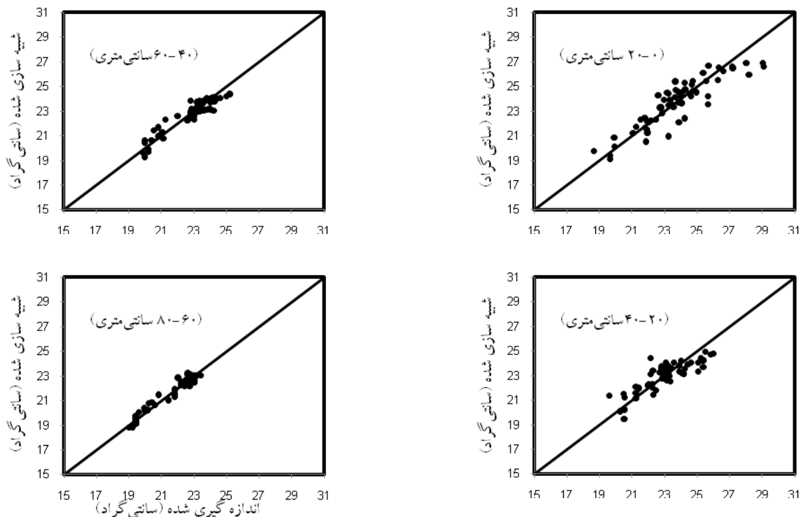
شکل ۲. مقایسه نتایج پیش‌بازی میانگین روزانه دمای خاک با مدل رگرسیونی چندگانه نسبت به مقادیر واقعی ثبت‌شده در عمق‌های a. ۰ تا ۲۰، b. ۲۰ تا ۴۰، c. ۴۰ تا ۶۰ تا d. ۶۰ تا ۸۰ سانتی‌متری
