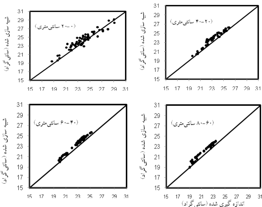
شکل ۱. مقایسه نتایج پیش‌بینی میانگین روزانه دمای خاک با مدل شبیه‌سازی COUP نسبت به مقادیر واقعی ثبت‌شده در عمق‌های a. ۲۰ تا ۰، b. ۲۰ تا ۴۰، c. ۴۰ تا ۶۰، d. ۶۰ تا ۸۰ سانتی‌متری
