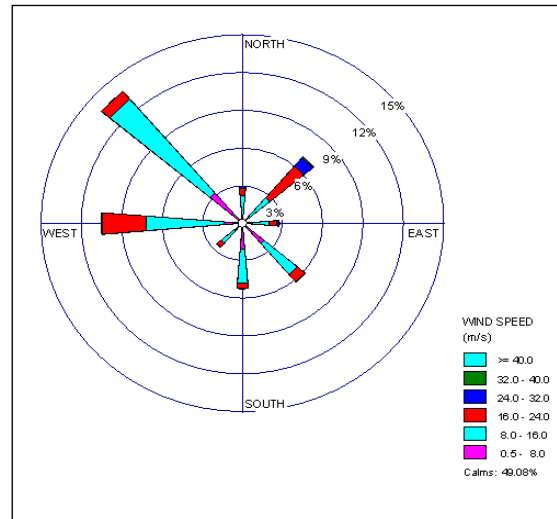
شکل ۳. گلباد سالانه‌ی ایستگاه روانسر (۱۹۹۷-۲۰۰۶)
