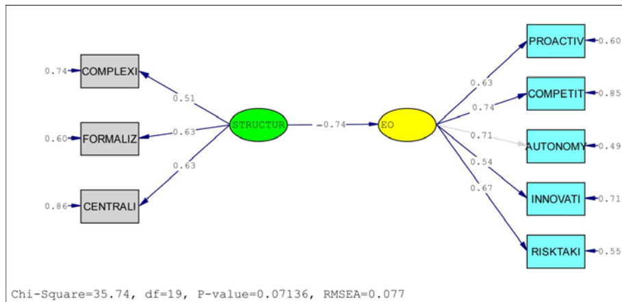
شکل (۳) - مدل معادلات ساختاری (ضرایب استاندارد شده)
