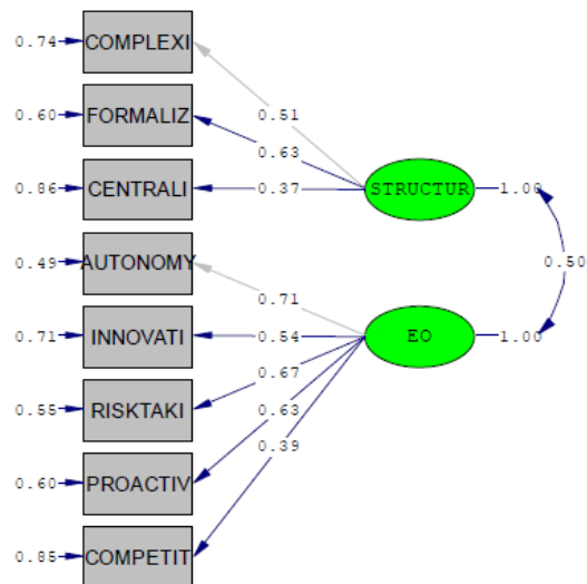
شکل (۲): مدل‌های اندازه‌گیری مربوط به دو سازه اصلی تحقیق
