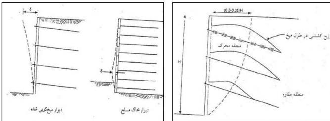
تصویر ۱۴- رفتار سیستم میخ کوبی. تصویر ۱۵- تفاوت تغییر مکان در دیوارهای خاک مسلح و دیوارهای میخ کوبی. (مأخذ: (دریا خاک و پی، ۱۳۸۰) (CLOUTERRE, 1991, 26)
