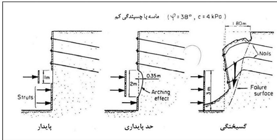
تصویر ۱۸- پایداری فازه‌های حفاری. مأخذ: (CLOUTERRE, 1991, 4)
