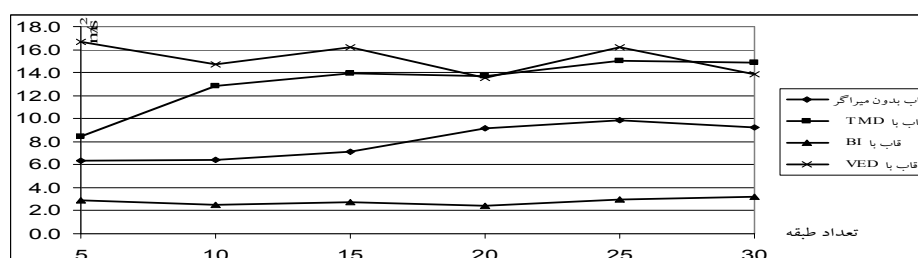
شکل (۱۰): شتاب حداکثر ایجاد شده در قاب‌ها تحت زلزله الاسترو
