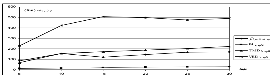
شکل (۹): برش پایه قاب‌ها تحت زلزله الاسترو
