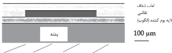
تصویر ۱- طرح شماتیک مقطع کلی بدنه‌های زیرلعابی. (۱) بدنه؛ (۲) لایه ظرف سفید بستر نقاشی (بوم‌کننده)؛ (۳) نقاشی؛ (۴) لعاب شفاف. ماخذ: (Voigt et al., 2006, 226)
