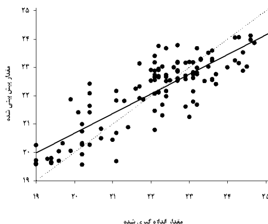
شکل ۸- نمودار پراکنش برای مقادیر مشاهداتی و شبیه سازی شده داده‌های آموزش آزمون در ANFIS
