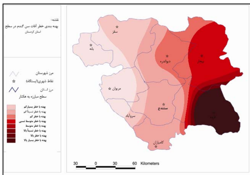
شکل ۲. پهنه‌بندی خطر آفت سن گندم در سطح استان کردستان
