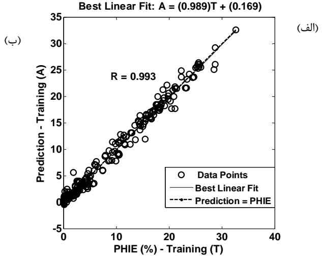
شکل ۱۱. نمودار همبستگی بین تخلخل و برآورد ترکیب آنسامبلی سه‌شبکه‌ای شبکه‌های ۱، ۲ و ۵ به روش خطی بهینه با استفاده از الگوریتم ژنتیک برای الف) الگوهای آموزش و ب) الگوهای آزمون.
