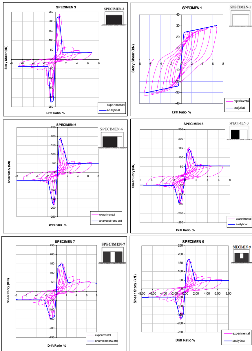
شکل ۵: مقایسه منحنی برش پایه در مقابل تغییر مکان با آنالیز و چرخه‌های هیستریزس نمونه‌های آزمایش شده [۸].
