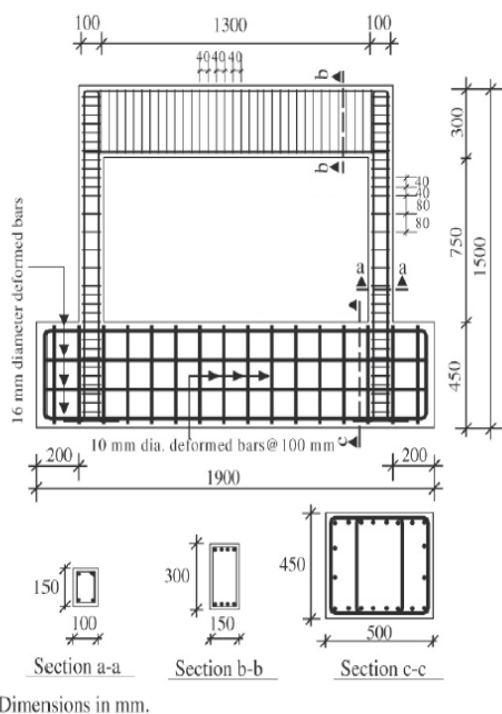
شکل ۱: ابعاد و جزئیات آرماتورگذاری قاب بدون میانقاب [۸].
