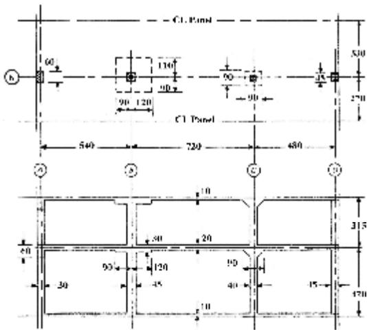
شکل ۹: سیستم دال تخت دوطرفه مثال ۲.
