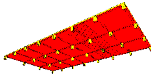
شکل ۸: سیستم صفحه تخت دوطرفه مورد تحلیل برای بررسی درستی عملکرد برنامه.
